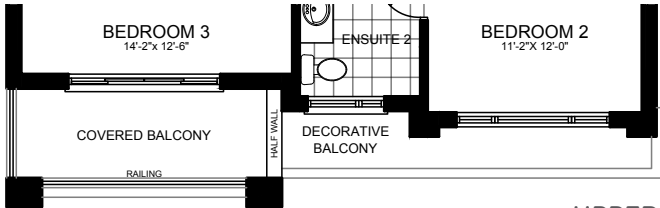
ELEV. C
