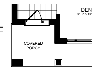
ELEV. C
