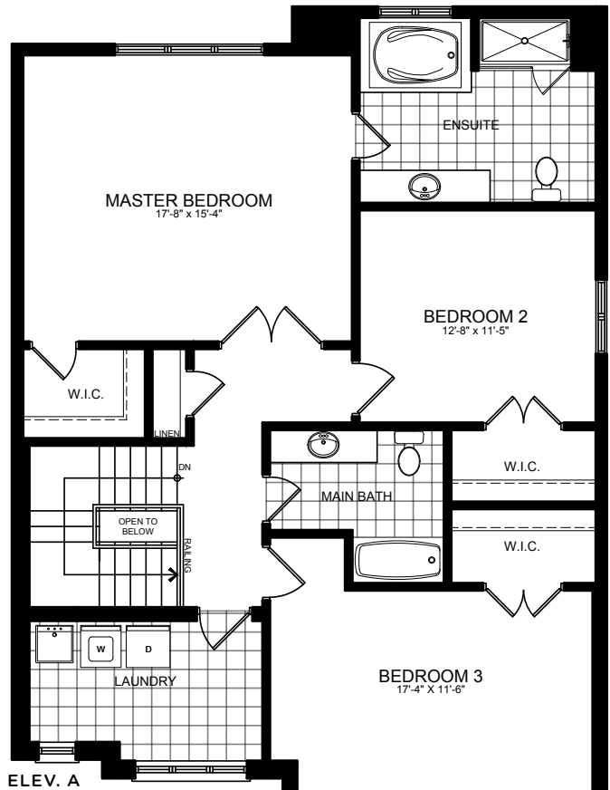
ELEV. A
