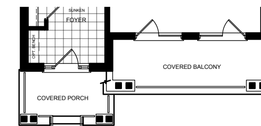
ELEV. B
