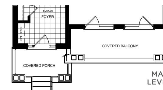
ELEV. C
