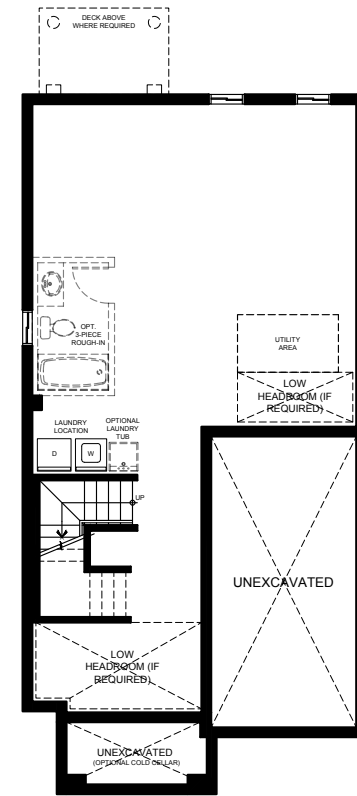
ELEV. A
