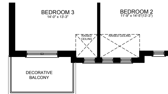
ELEV. B
