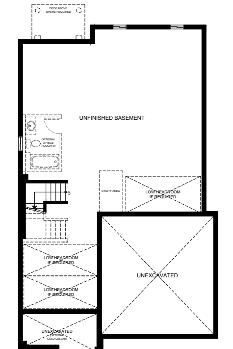
ELEV. A
